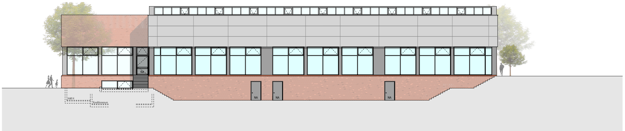
Nordwestansicht
