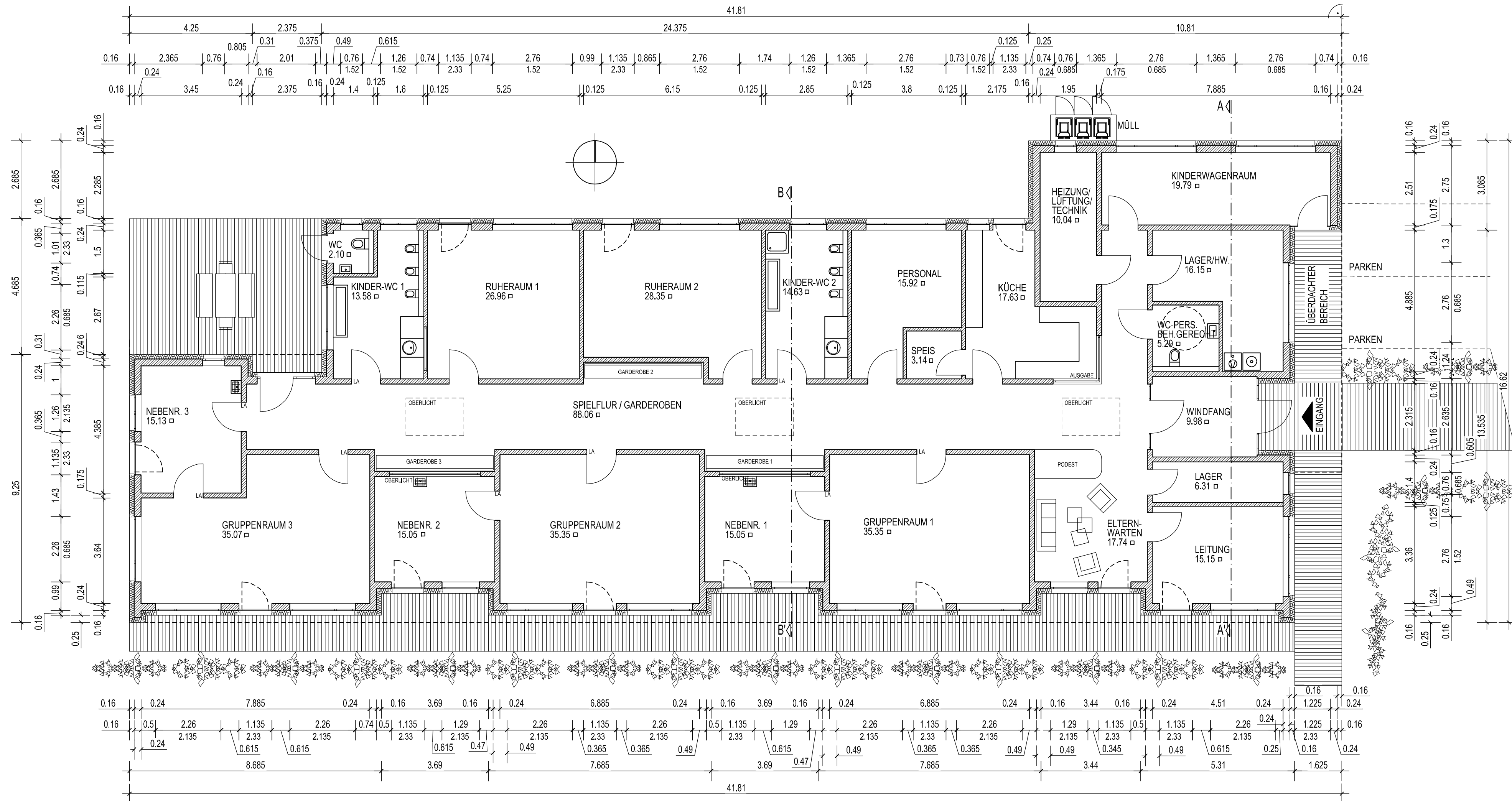
ERDGESCHOSS 1:100
